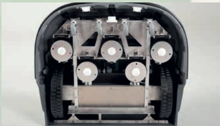
Unteransicht: 5 Schneidköpfe
